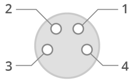
Cable side
